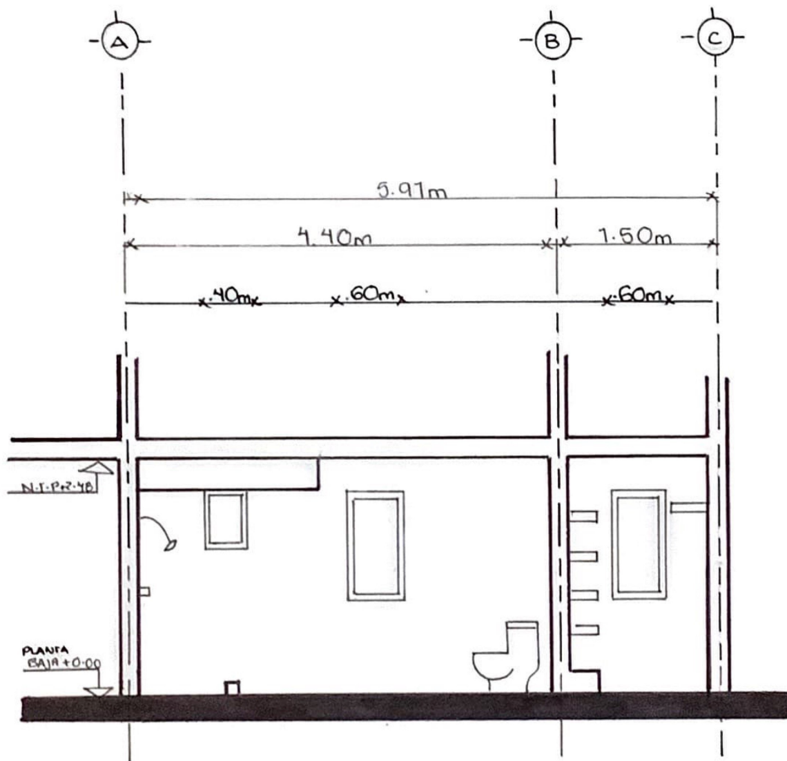
CORTE C-C' TRANSVERSAL ESCALA - 1:50
