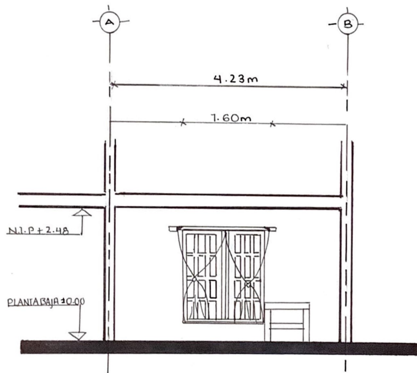
CORTE A-A' TRANSVERSAL ESCALA — 1:50
