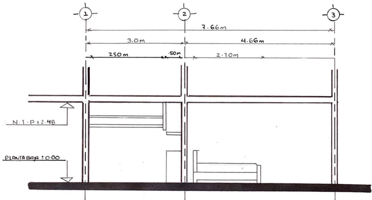
CORTE B-B' LONGITUDINAL ESCALA - 1:50
